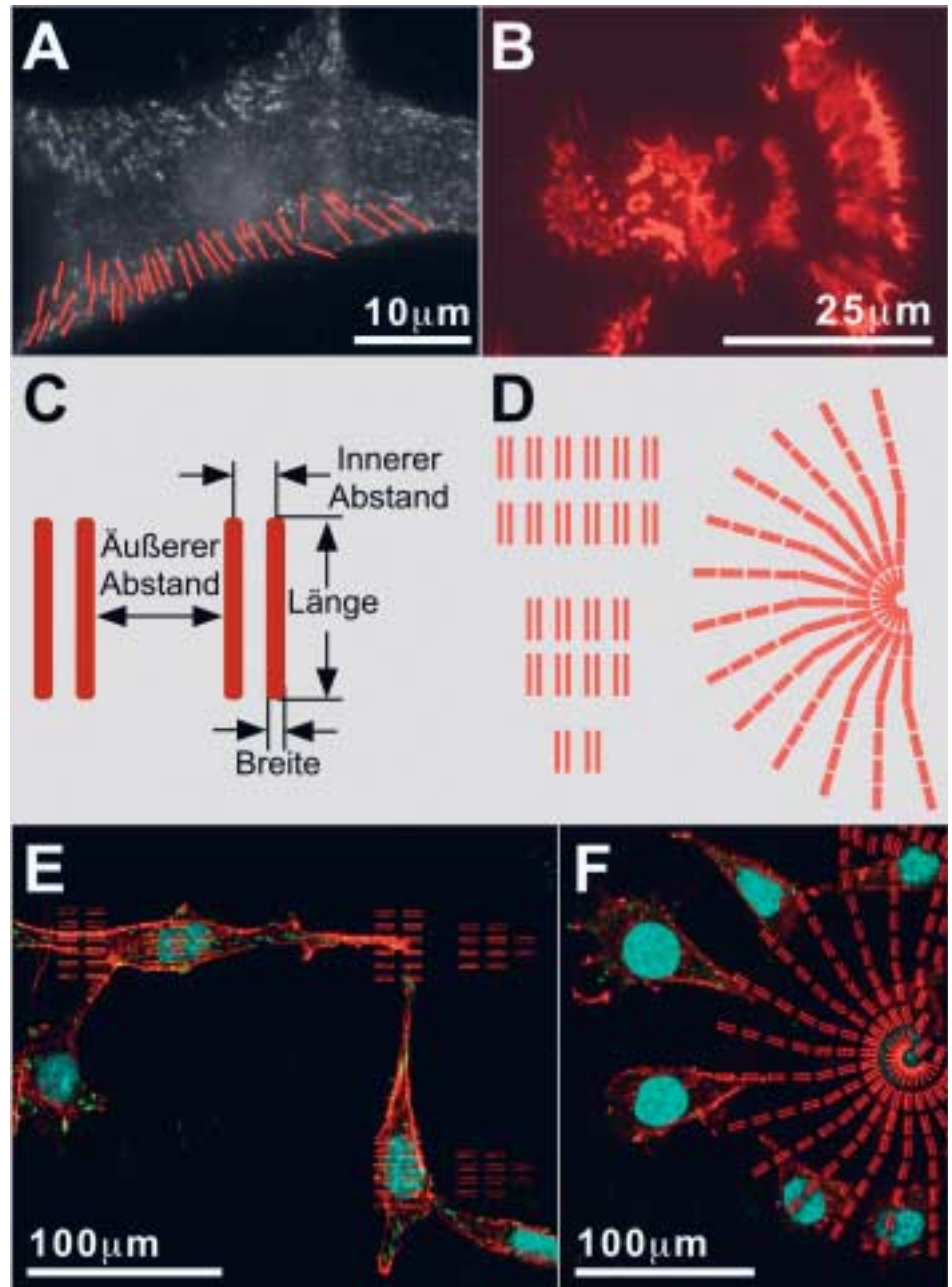
Abbildung 1 A zeigt unter Eiweißmangel gehaltene Bindegewebszelle mit ausgeprägter Substrathftung. Die Fokale Adhäsionskinase wurde mit einem fluoreszenzmarkiertem Antikörper angefärbt und mittels TIRF-Mikroskopie abgebildet. Die in rot hervorgehobenen Strukturen geben die Dimensionen für das in Abbildung 1C abgebildete Design der Haftstreifen. Abbildung 1 B zeigt ein typisches Haftmuster einer Bindegewebszelle nach Färbung des direkt am Glaskontakt liegenden Aktin-Zytoskeletts mittels TIRF-Mikroskopie. Einer halbmondförmigen Haftregion im vorderen Zellteil (rechts) folgt ein zentraler Bereich mit Punkthaftung (links). Abbildungen 1 C und D geben ein Beispiel für die Anordnung der Streifen zu größeren Strukturgruppen nach dem Vorbild des Haftmusters der Bindegewebszelle und alternativ als Halbkreis ("Rosette"). In den Abbildungen 1 E und F ist die zellausrichtende Wirkung der Strukturen zu erkennen. Bindegewebszellen entwickeln eine Spindelform und spannen sich zwischen den Strukturgruppen auf (links). Die Rückseiten desselben Zelltyps werden von der Rosettenstruktur gebunden und die Zellen richten sich kranzförmig aus.
